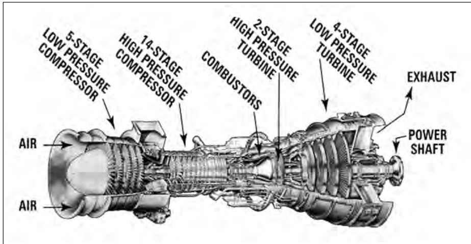
Figura 1. Este gráfico de una LM2500 explica tan bien el principio de trabajo de una turbina de gas que no son necesarias más explicaciones.
